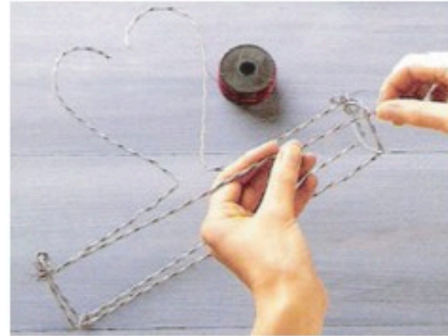
الشكل ( ٩٩ )
